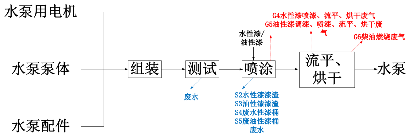
图 2-7 项目水泵生产工艺流程图
