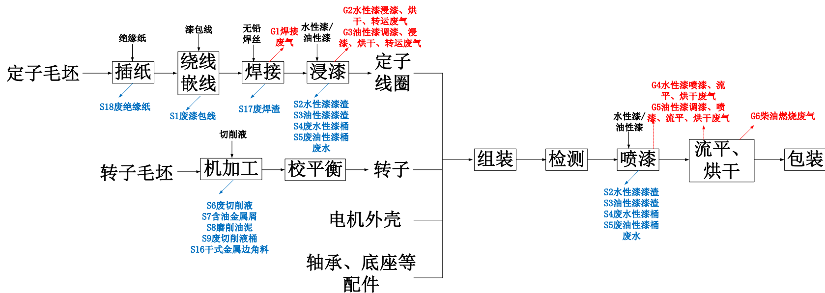
图 2-6 项目电机生产工艺流程图
