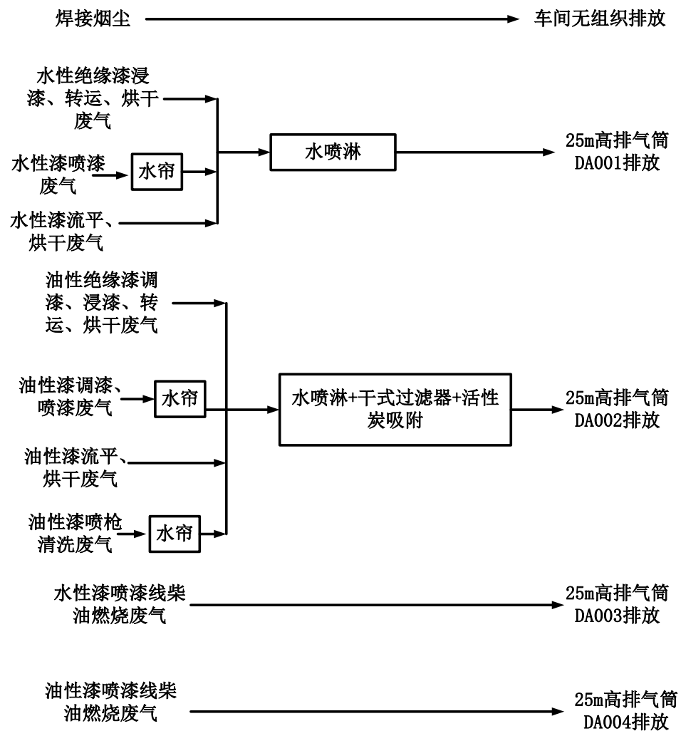
图 4-1 项目废气治理工艺流程图
