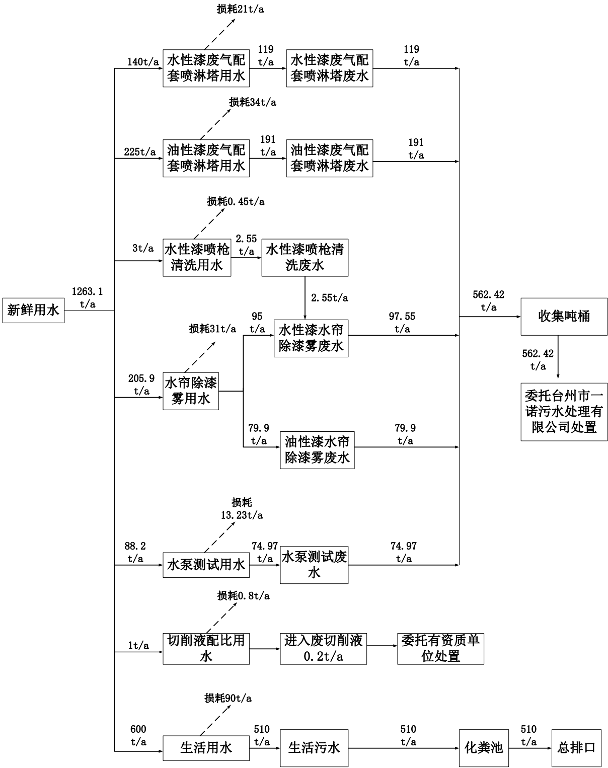
图 2-1 项目水平衡图 单位：t/a
