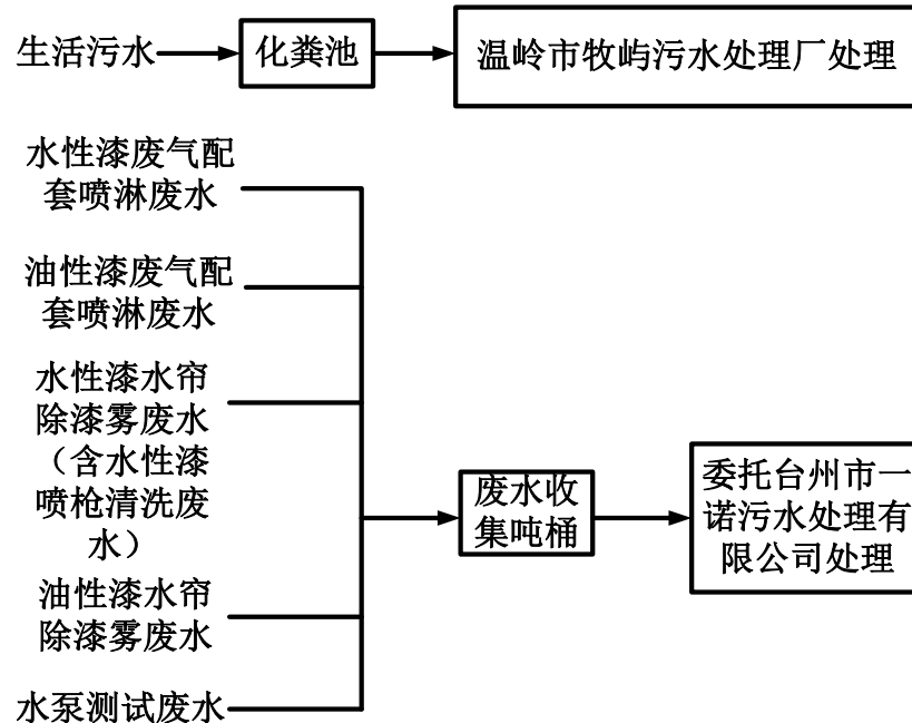
图 4-2 项目废水处理工艺流程图
