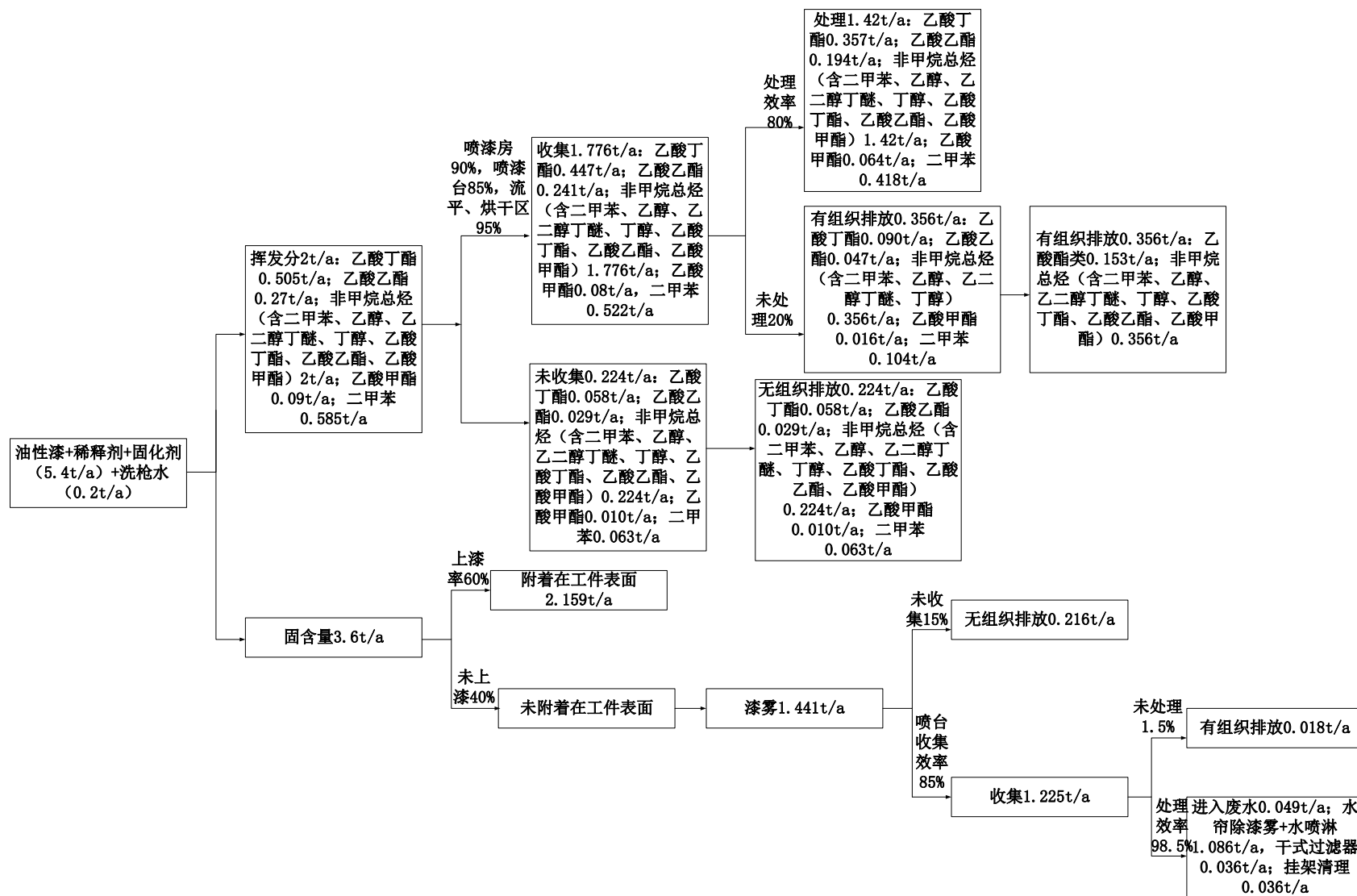
图 2-2 项目油性漆（包含稀释剂、固化剂）物料平衡图
