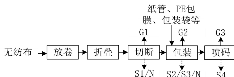
图 2-2 干巾、面膜布、抹布卷工艺流程及污染物产生节点图
