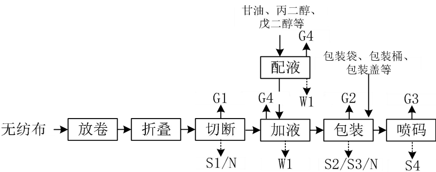
图 2-3 湿巾工艺流程及污染物产生节点图
